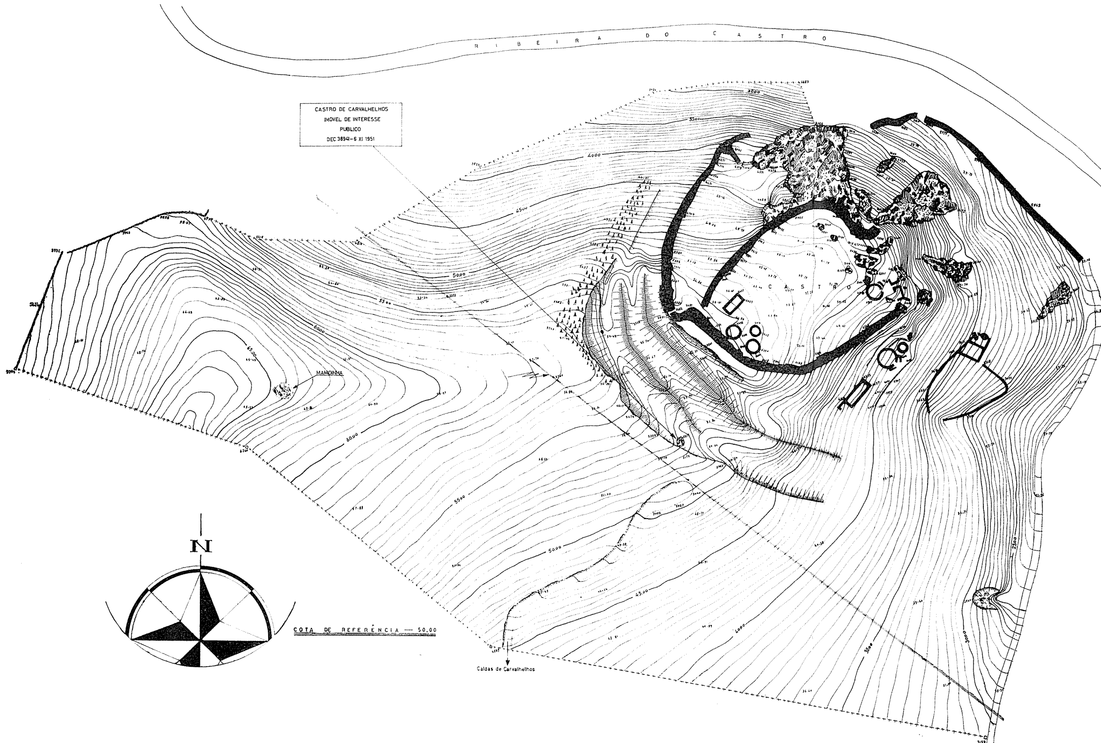
Fig. 1 — Planta do Castro de Carvalhelhos e da zona de protecção cedida pela Direcção-Geral dos Serviços Florestais e Aquícolas (Ministério da Economia). O desenho da planta pelo qual se fez esta gravura foi feito pelo Sr. Dr. Ascenso Metelo na escala 1/500. Com a redução na gravura a escala desta é, aproximadamente, 1/1130.
