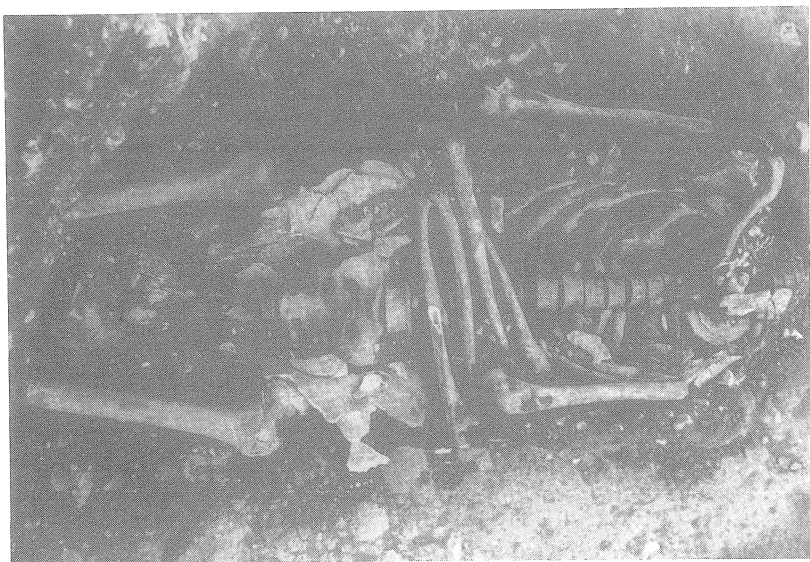
Fig. 5 — Esqueleto masculino encontrado no Forum. Séc. V d. C.
