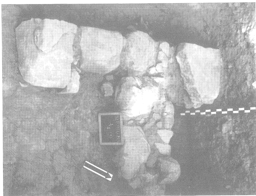
Fig. 6 — Alicercas romanos aproveitados para enterramentos de inumação - A1 (3). Post. D. Afonso III.
